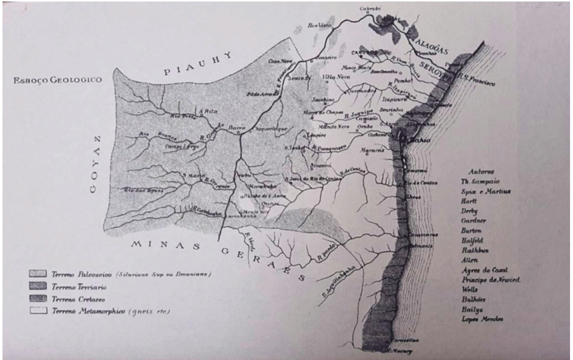
Figura 1- Esboço Geológico do Estado da Bahia
